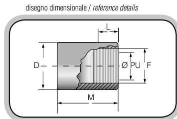
disegno dimensionale / reference details
